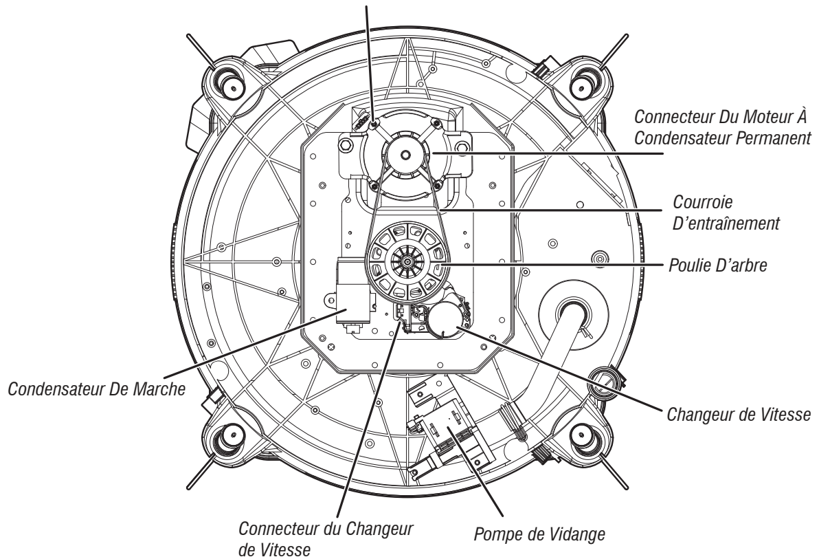
Illustration 8 – Vue du bas – COND PERM
