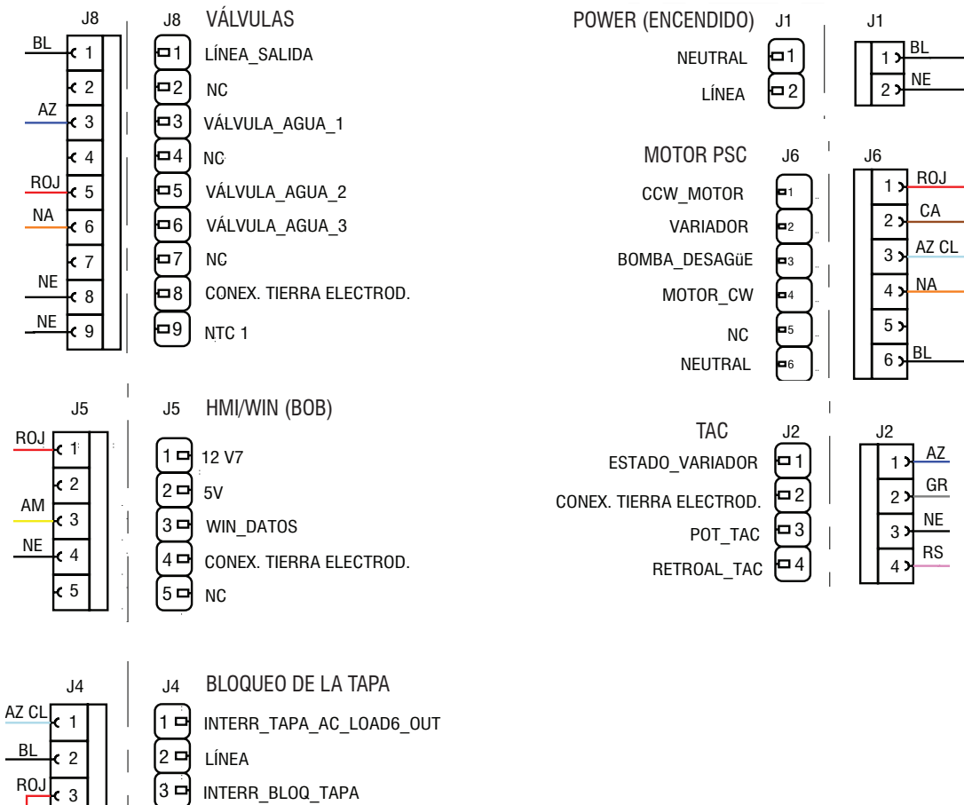
Figura 5: Conector y patillas
